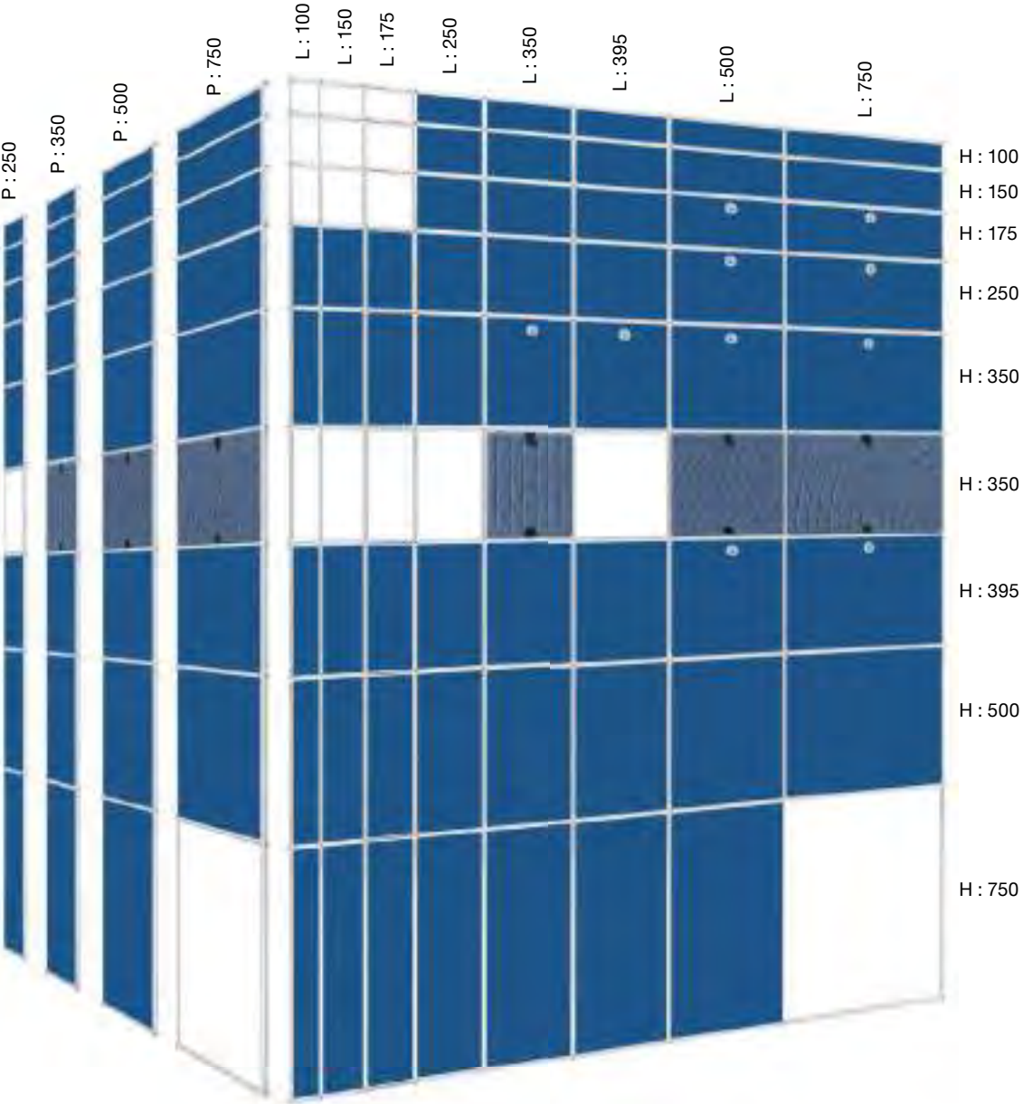
Toutes les dimensions sont en mm.
